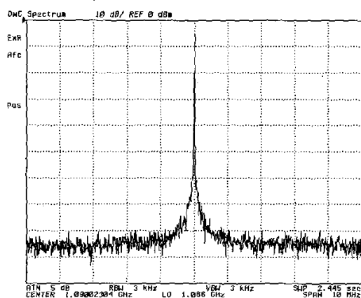
Fig. 6. Output spectrum.
